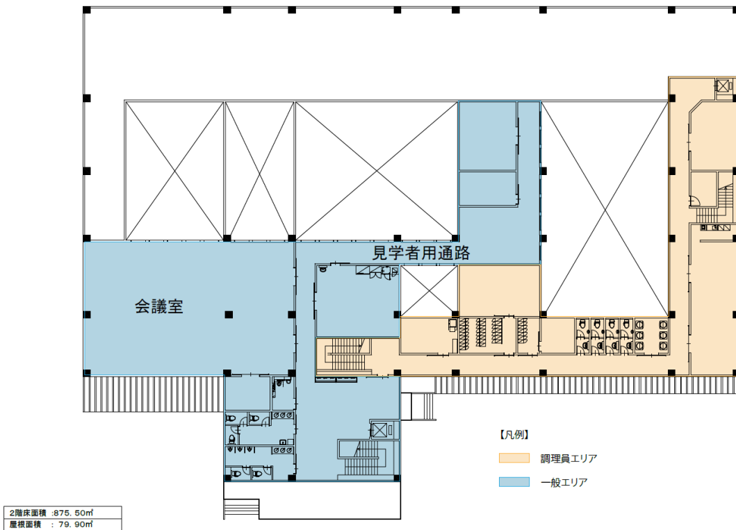
図 4-5 平面図 (2F)
