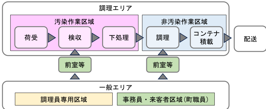
図 3-3 作業動線の考え方
