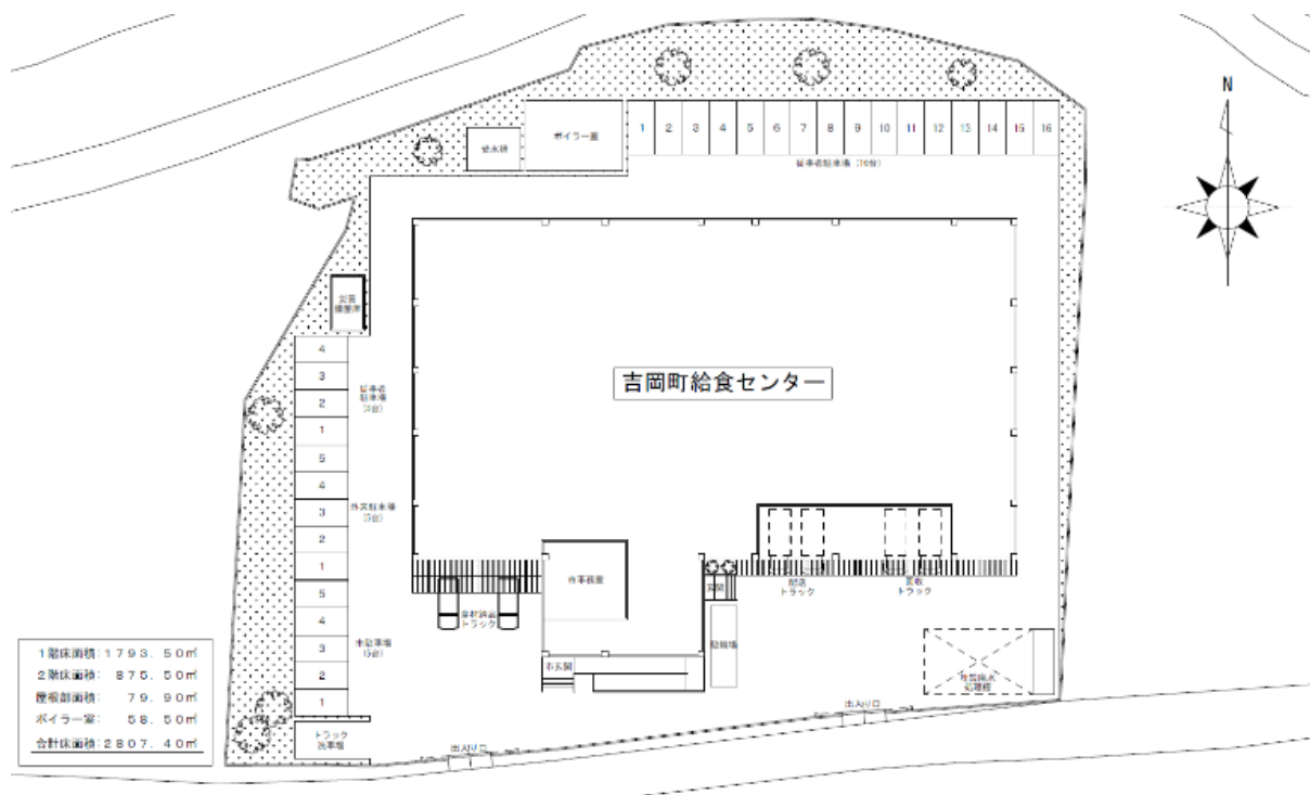
図 4-3 配置図
