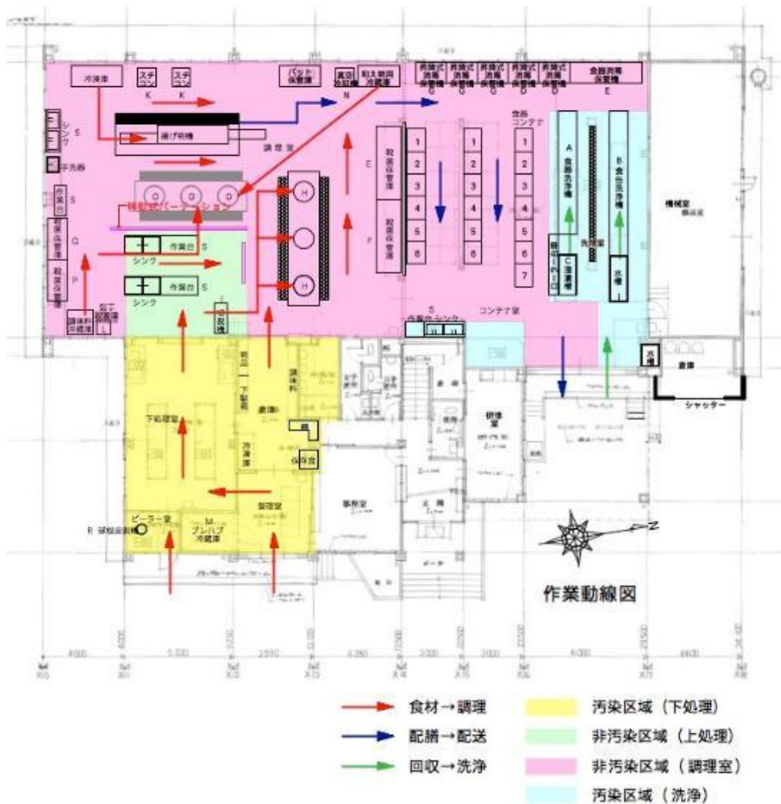
図 1-4 現施設の作業動線図
