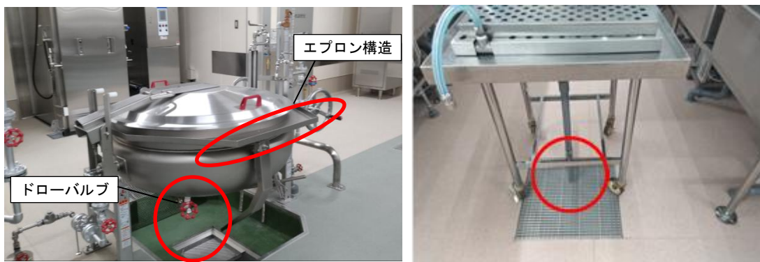
図 3-4 ドライ仕様の回転釜
